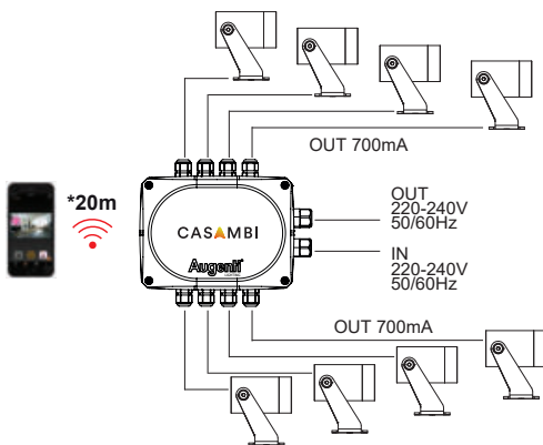
Bloom Mini HUB.700.001.CA 700mA CASAMBI MAX 8 pz.
